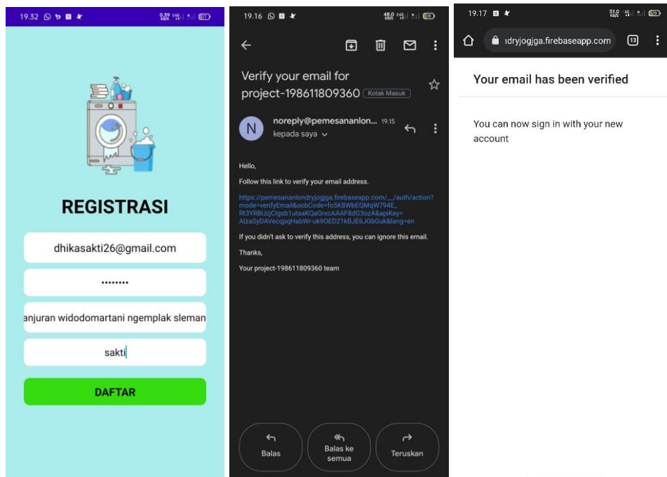
tampilan registrasi
